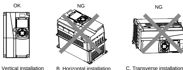
Рис 4.1 Установка ПЧ
