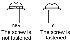
Рис 4.17 Правильная установка винтов
