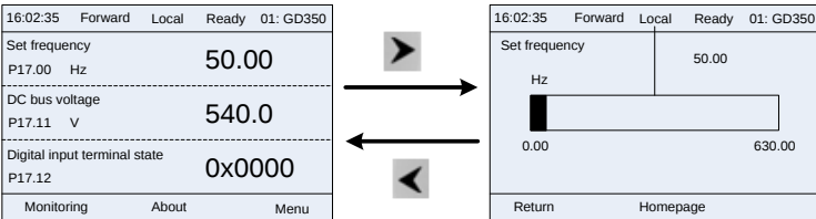
Рис 5.4 Отображение параметров при останове ПЧ
