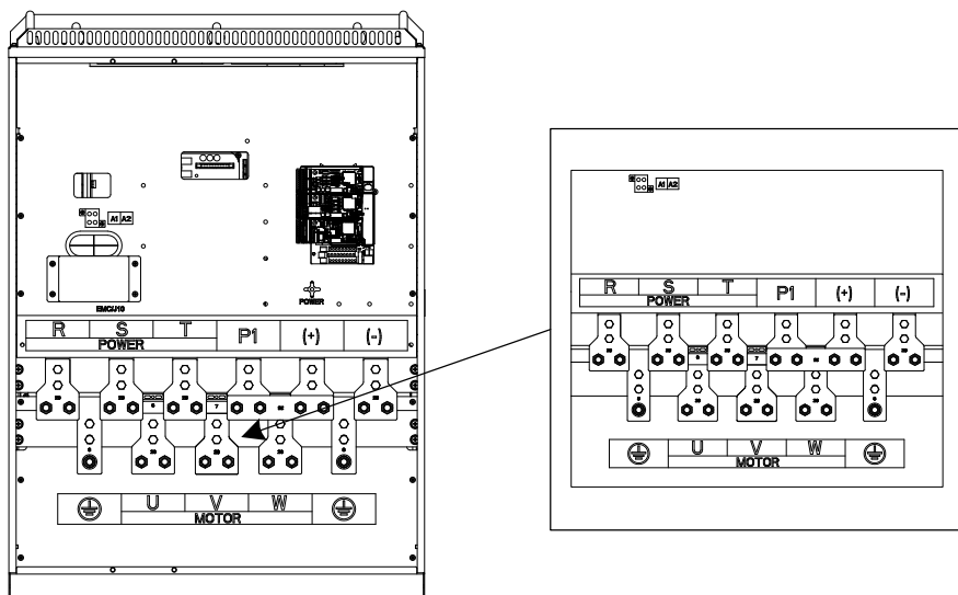
Рис 4.15 Клеммы силовых цепей 380 В 220–315 кВт и 660 В 250–355 кВт
