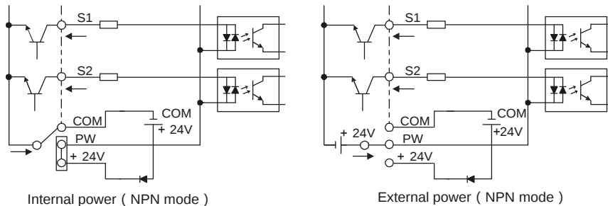
Рис 4.20 NPN режим
