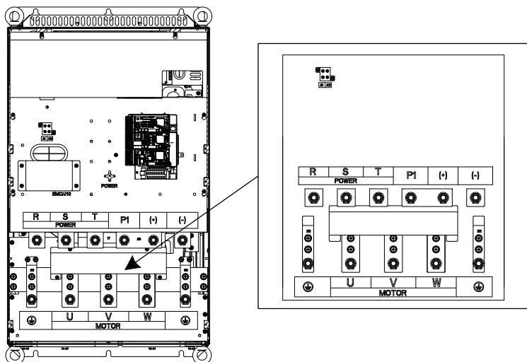
Рис 4.14 Клеммы силовых цепей 380 В 132–200 кВт и 660 В 160–220 кВт
