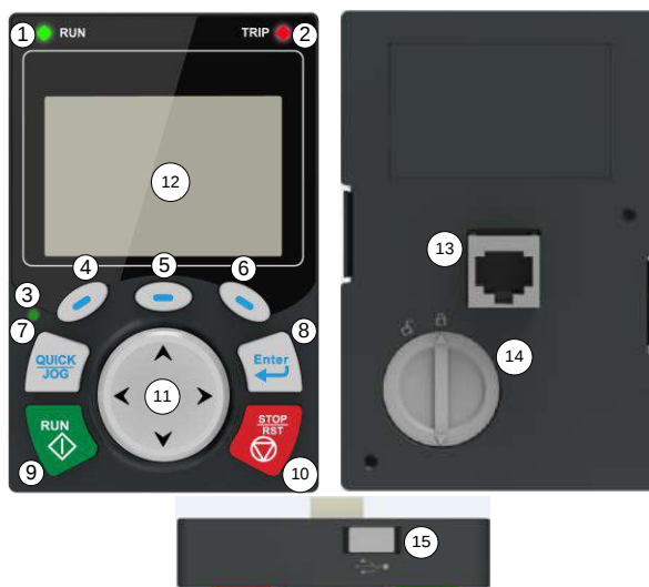
Рис 5.1 Панель управления (внешний вид)
