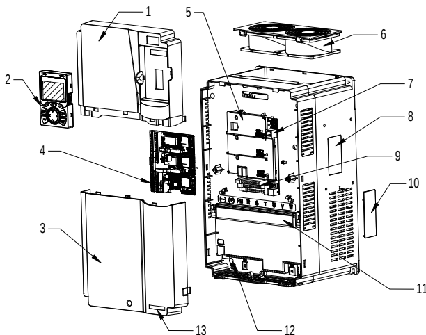
Рис 3.7 Структурная схема
