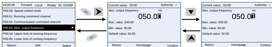
Рис 5.16 Интерфейс редактирования параметров
