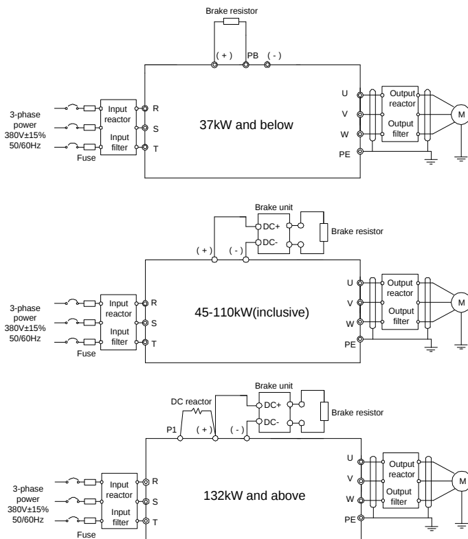
Рис 4.7 Схема подключения силовой цепи 380 В(-15%)–440 В(+10%)
