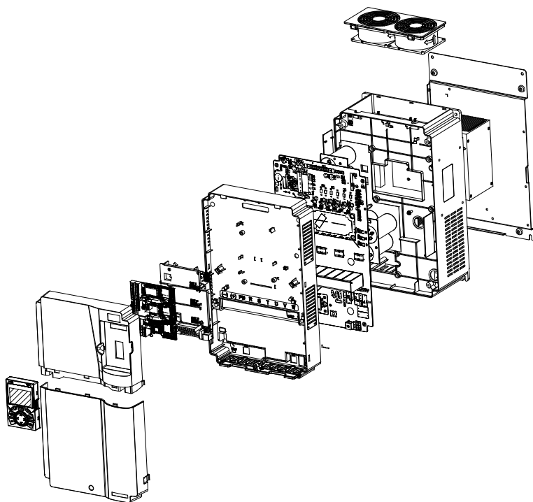
Рис 0.3 Структура ПЧ
