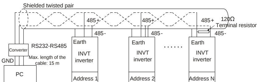
Рис 9.4 Практическая схема
