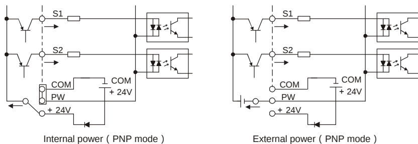
Рис 4.21 PNP режим
