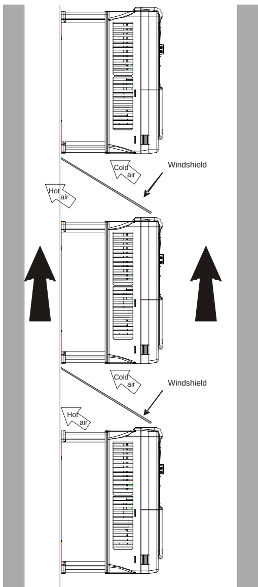
Рис 4.5 Вертикальная установка
